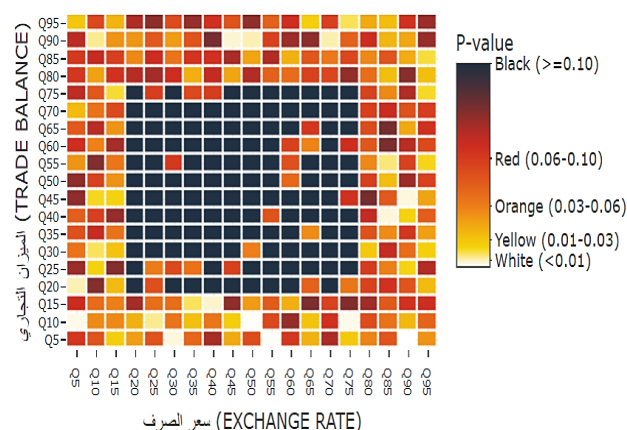
شكل رقم (8): اختبار السببية عبر Quantiles
