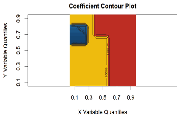
شكل رقم (12): خريطة الخطوط الكنتورية لمعاملات الأثر (Coefficient Contour Plot)
